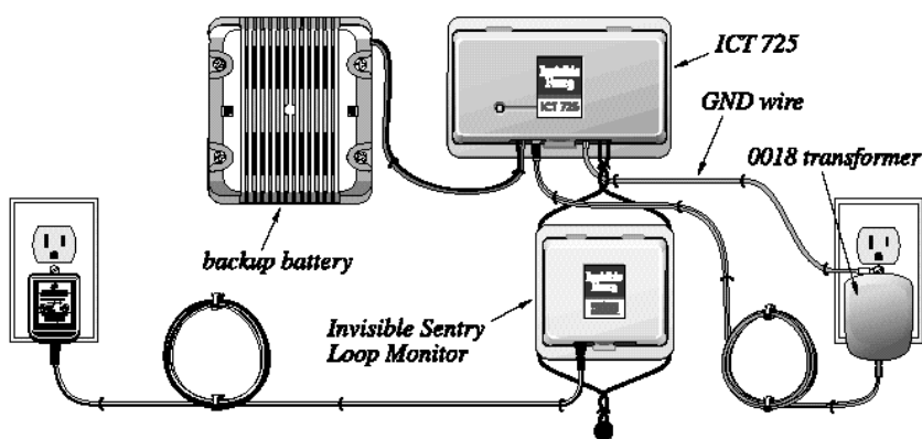
Système ICT 725 avec batterie de secours et système Invisible Sentry MC .
